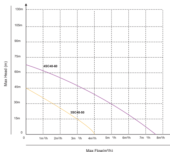
流速曲线
