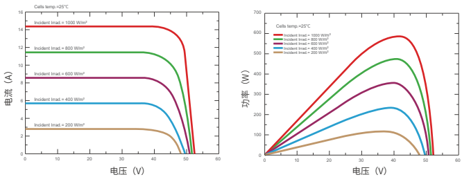
电流电压及功率电压曲线 (SKT590M10)
