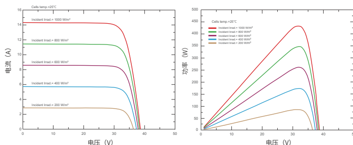
电流电压及功率电压曲线 (SKT430M10-108D4)
