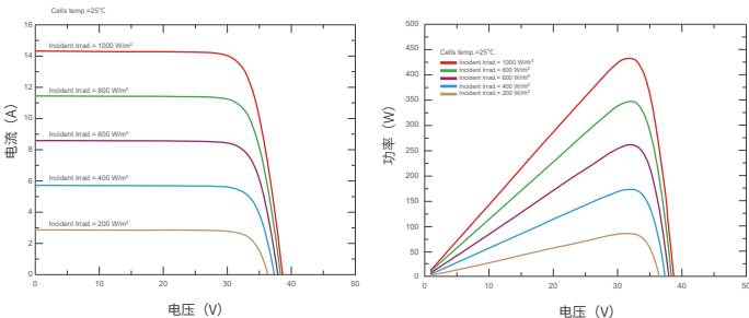
电流电压及功率电压曲线 (SKT430M10-108S3)
