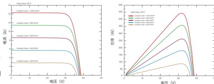
电流电压及功率电压曲线 (SKT440M10-108D4)
