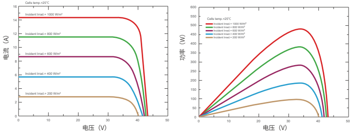
电流电压及功率电压曲线 (SKT480M10-120D5)
