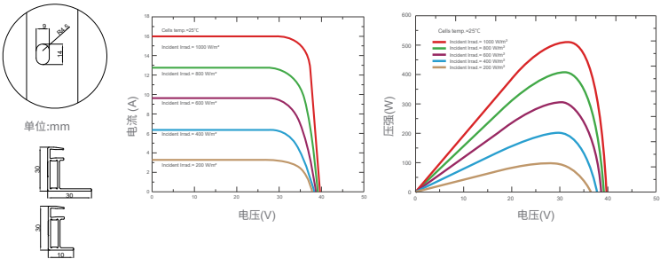
电流电压及功率电压曲线 (SKT510M12-108D4)
