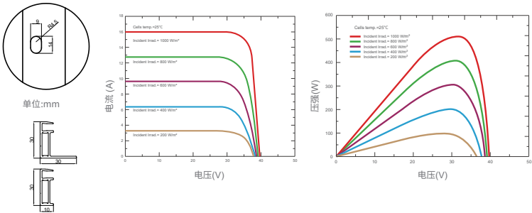
电流电压及功率电压曲线 (SKT510M12-108D5)
