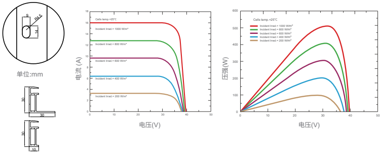
电流电压及功率电压曲线 (SKT510M12-108D6)
