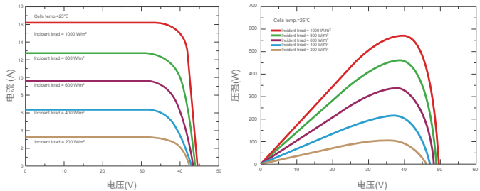
电流电压及功率电压曲线 (SKT565M12-120D5)
