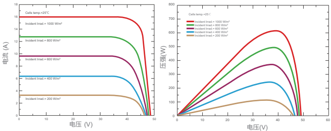
电流电压及功率电压曲线 (SKT620M12-132D3)
