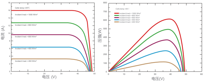
电流电压及功率电压曲线 (SKT620M12-132D5)
