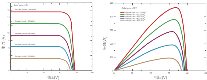
电流电压及功率电压曲线 (SKT460M12-96D6)
