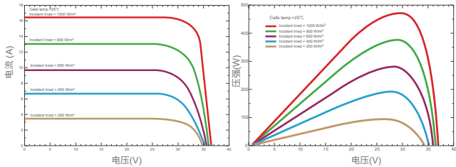
电流电压及功率电压曲线 (SKT470M12-96D5)
