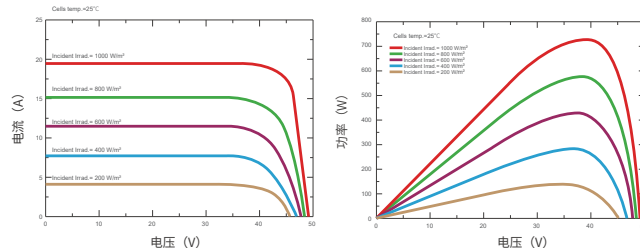
电流电压及功率电压曲线 (SKT730M12-132D4)
