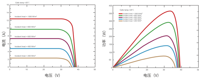
电流电压及功率电压曲线 (SKT370M10)
