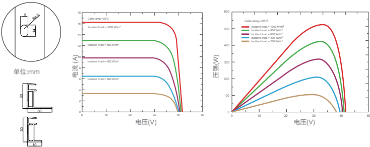
电流电压及功率电压曲线 (SKT525M12-108D4)
