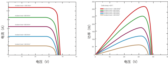
电流电压及功率电压曲线 (SKT330M10)
