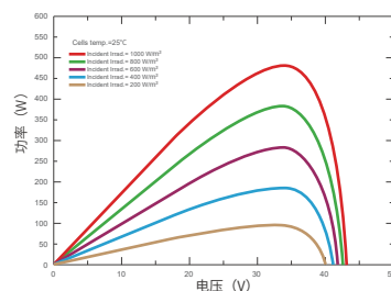
电流电压及功率电压曲线 (SKT480M10-120D4)
