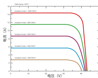
电流电压及功率电压曲线 (SKT480M10-120D4)
