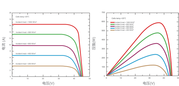
电流电压及功率电压曲线 (SKT585M12-120D5)
