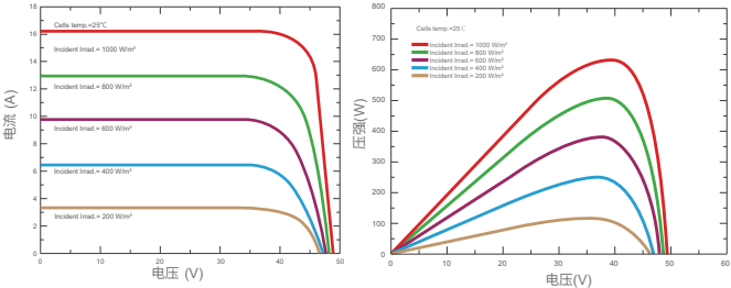
电流电压及功率电压曲线 (SKT630M12-132D5)
