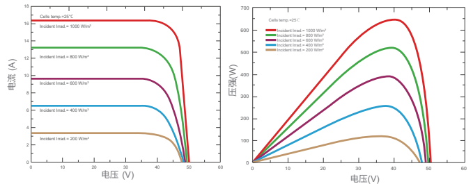
电流电压及功率电压曲线 (SKT645M12-132D5)
