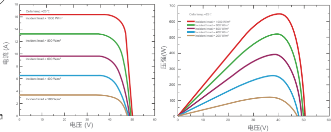
电流电压及功率电压曲线 (SKT645M12-132D3)
