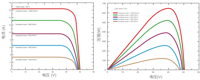
电流电压及功率电压曲线 (SKT645M12-132D4)
