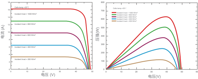
电流电压及功率电压曲线 (SKT630M12-132D4)
