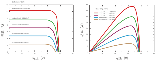
电流电压及功率电压曲线 (SKT375M10)
