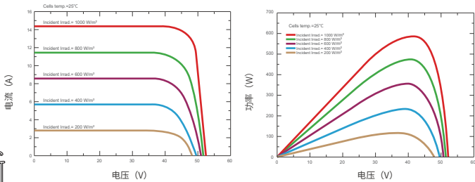
电流电压及功率电压曲线 (SKT590M10-144D5)
