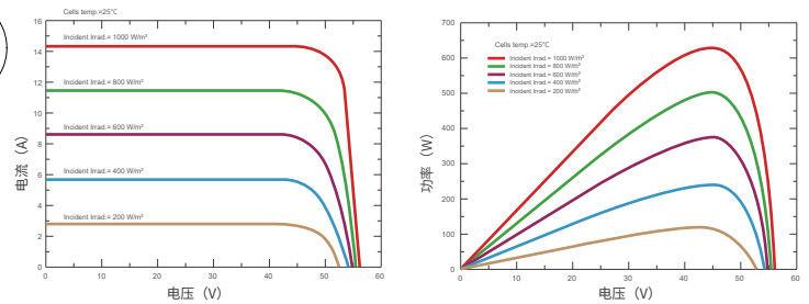
电流电压及功率电压曲线 (SKT625M10-156D4)
