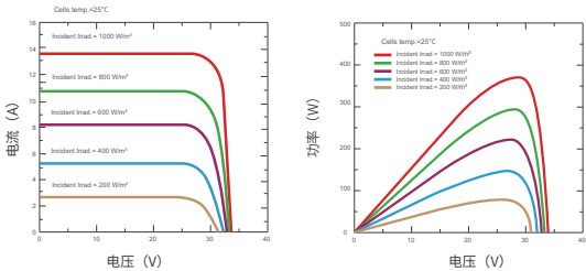
电流电压及功率电压曲线（SKT370M10）
