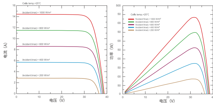
电流电压及功率电压曲线 (SKT435M10-108S3)
