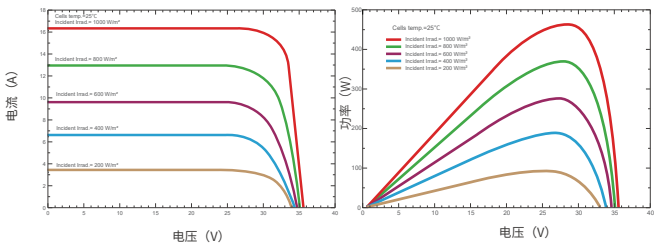
电流电压及功率电压曲线 (SKT460M10)
